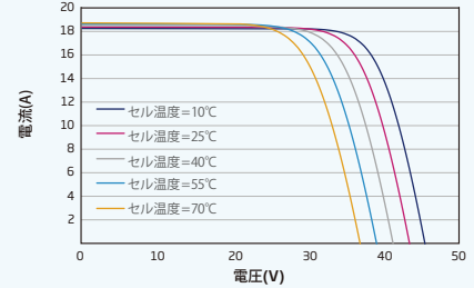
PVモジュール(650W)のI-V曲線
