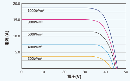
PVモジュール(650W)のP-V曲線
